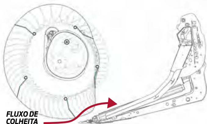
Posição 1 do excêntrico
