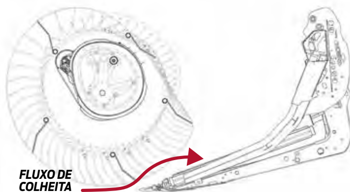
Posição 4 do excêntrico
